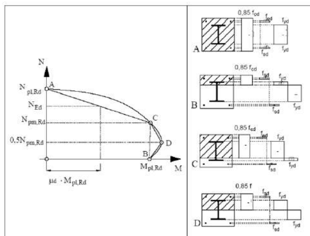
Figura 4.3.8 - Metodo semplificato per la valutazione del dominio di interazione N-M per le colonne composte
